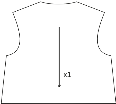
Trasero T.B Sastrero Talle: M Chaqueta conjunto Art. nº0-105
